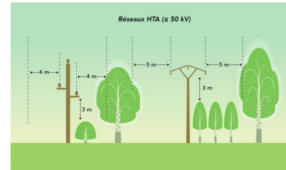
Isolateurs rigides.
